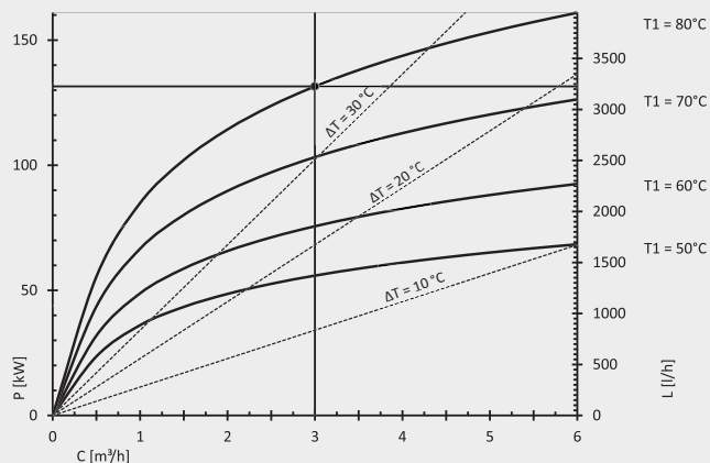
Wykres wydajności Storatherm Aqua Heat Pump 500/1 dla temperatury odbioru 45 °C
